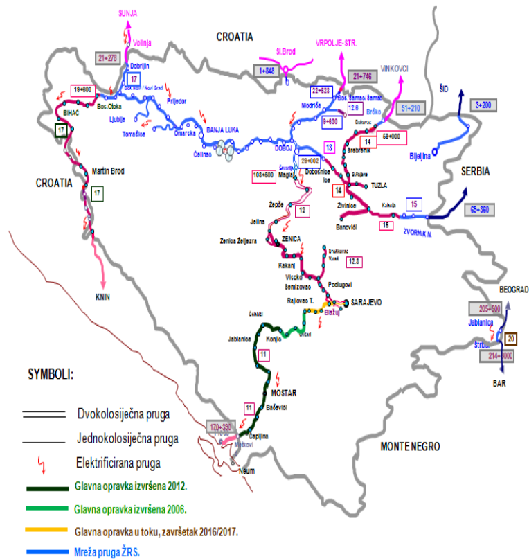
Karta 8 Radovi na željezničkoj mreži u FBiH (Izvor: ŽFBiH)
