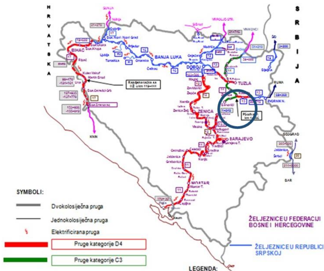
Karta 6 Željeznička mreža u BiH i FBiH, kategorizacija ŽFBiH (Izvor: ŽFBiH)
